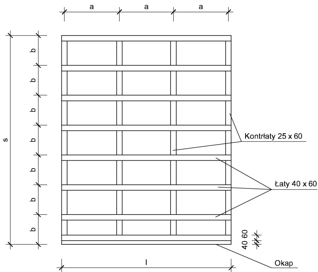
Rysunek 3. Układ kontrłat i łat
