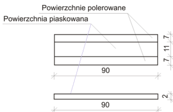
Rysunek roboczy pręgu kamiennego. Przykładowe wymiary w [cm].
