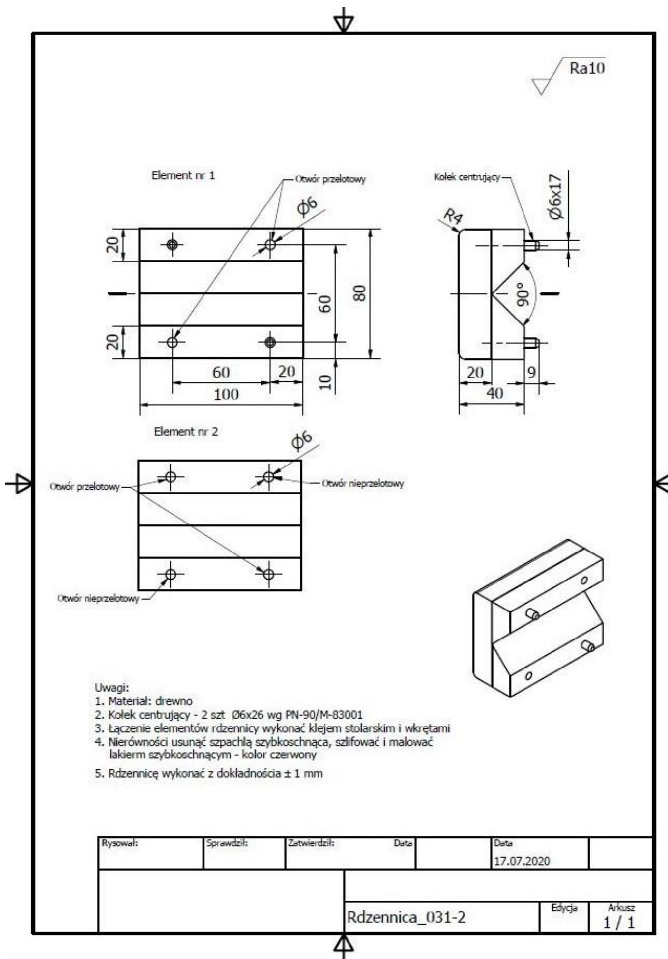
Rysunek 1. Rysunek wykonawczy rdzennicy
