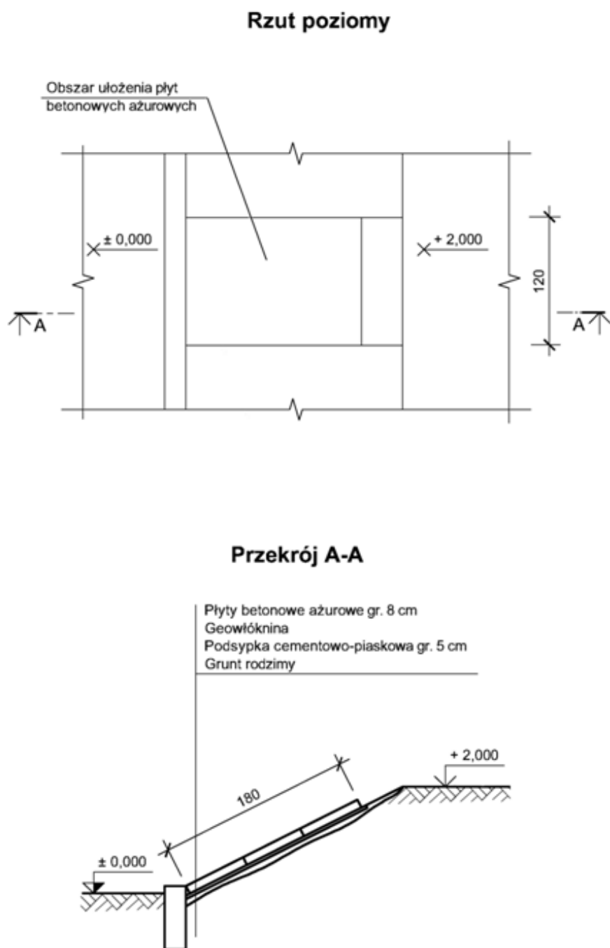
Rysunek 1. Fragment umocnienia skarpy
