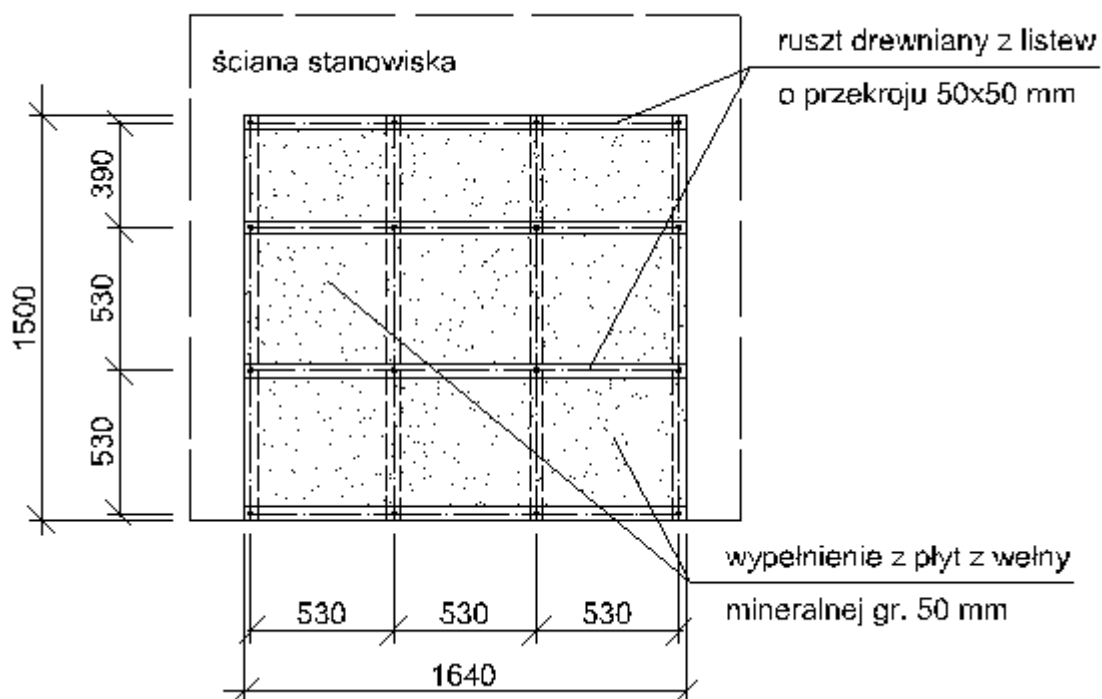
Rysunek 2. Ruszt poziomy i wypełnienie z płyt z wełny mineralnej
