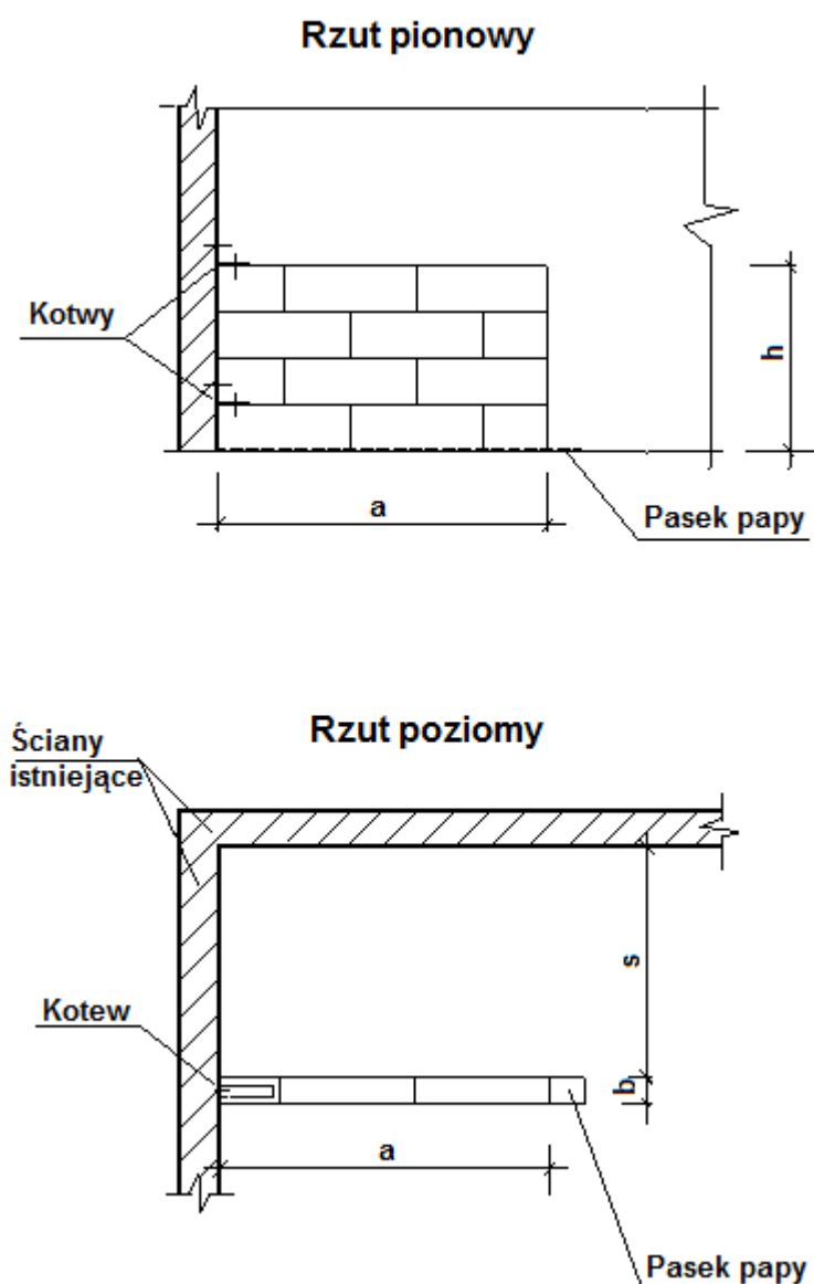
Rysunek 1. Fragment ścianki działowej
