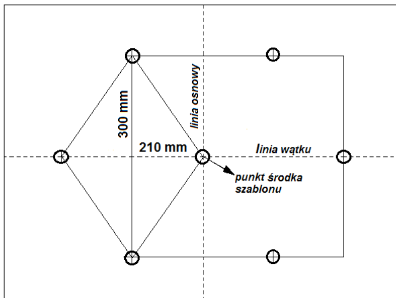
Rys. 2. Szablon pomocniczy z wyrysowanym podziałem przeszyc rombu wielokrotnego.
