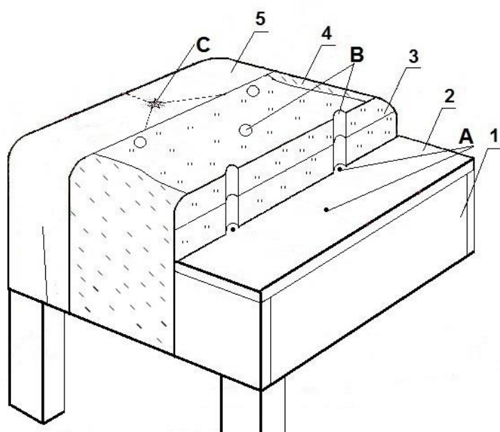
Rys. 1. Przekrój tapicerowanego podnóżka.
