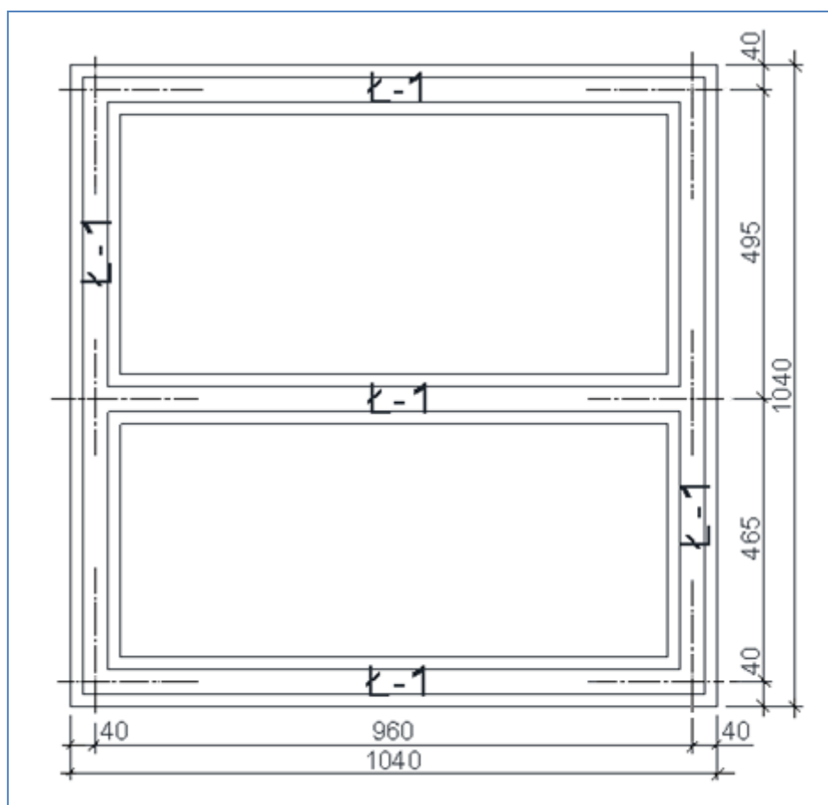
Rysunek 1. Rzut ław fundamentowych
