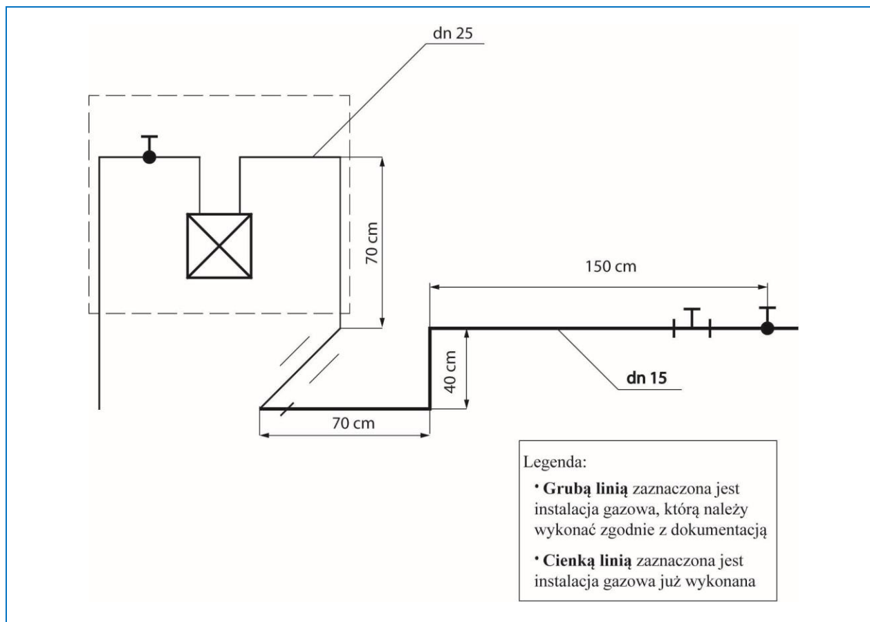
Rysunek 2. Rzut aksonometryczny przewodów instalacji gazowej w budynku jednorodzinnym
