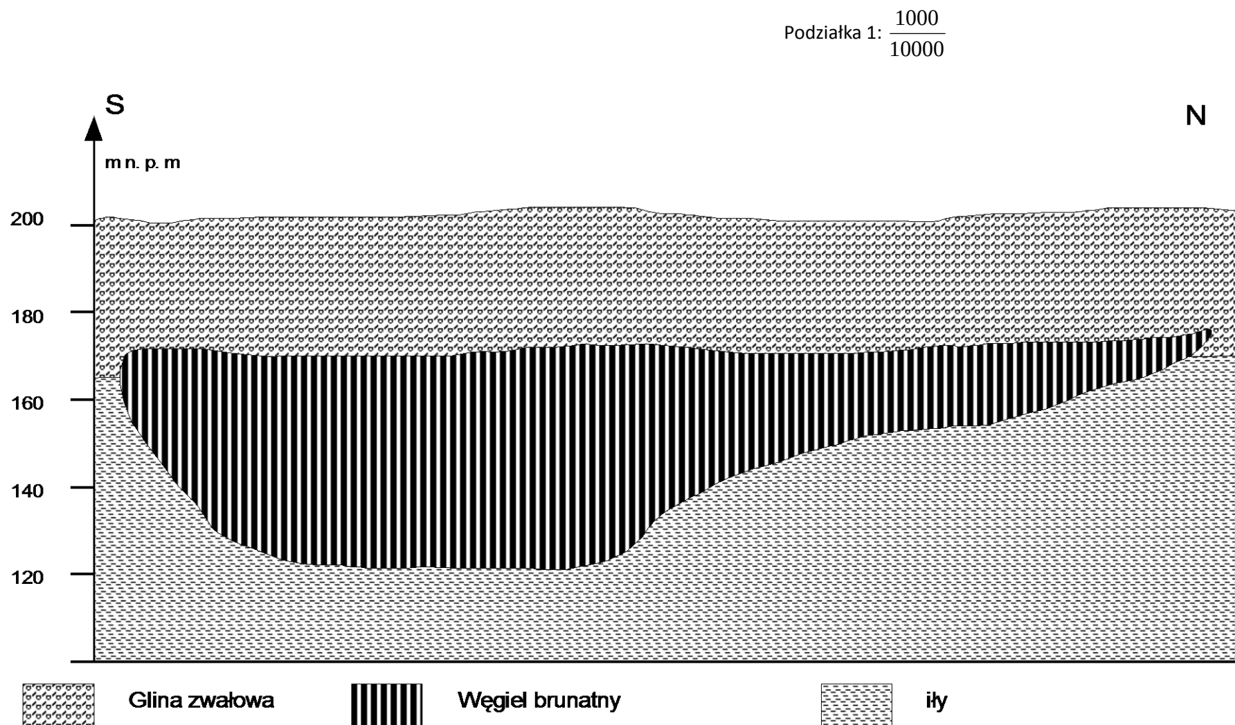
Rysunek nr 2 . Przekrój geologiczny A-A przez złożo „Marianek”
