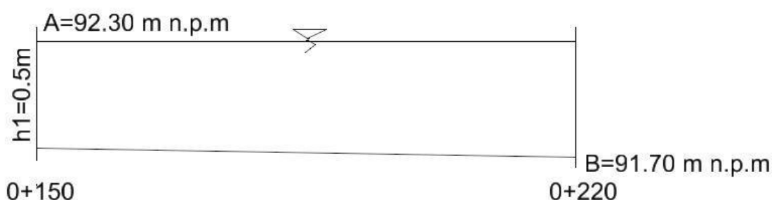
Rysunek. Spadek dna rowu melioracyjnego
