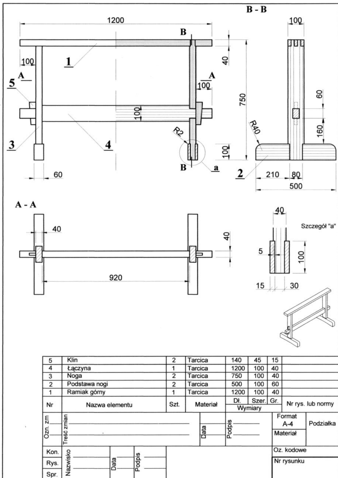
Rysunek stojaka
