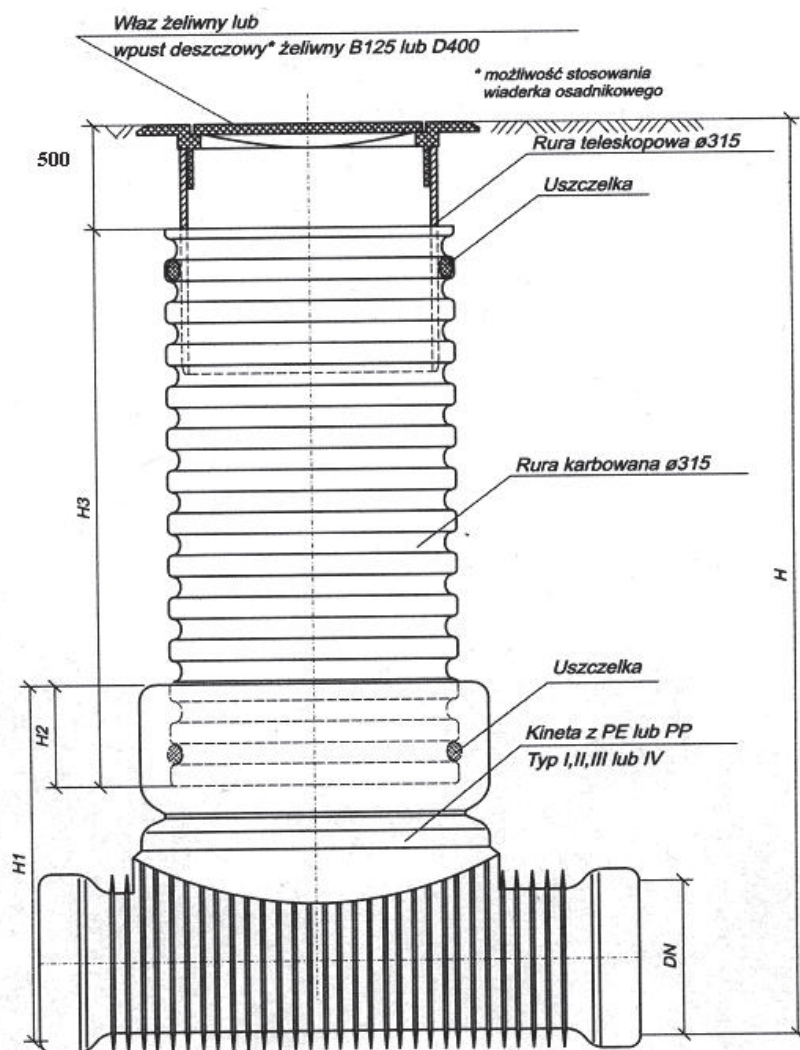
Rysunek 2. Studzienka kanalizacyjna Ø315 z włazem lub wpustem żeliwnym
