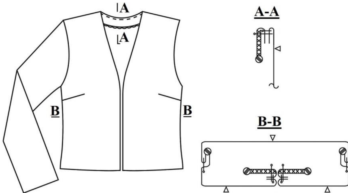
Rys. 2. Rysunek strukturalny wdzianka
