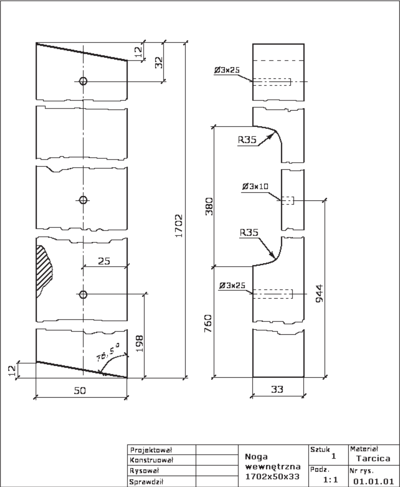
Rysunek nogi wewnętrznej
