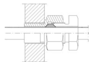
czujnik prosty TER-P-K-J/K-07 z uchwytem zaciskowym UZG-47
