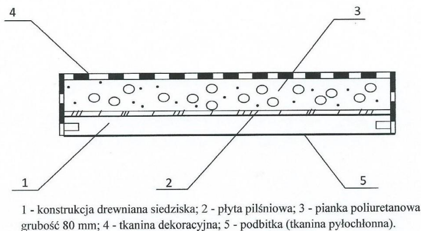
Rys. 1. Przekrój siedziska fotela
