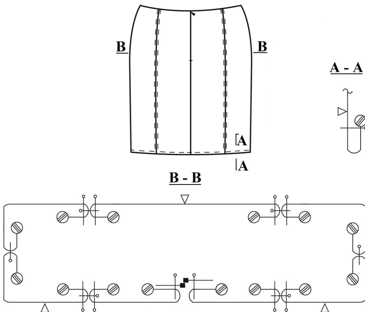
Rysunek 2. Schemat strukturalny spódnicy
