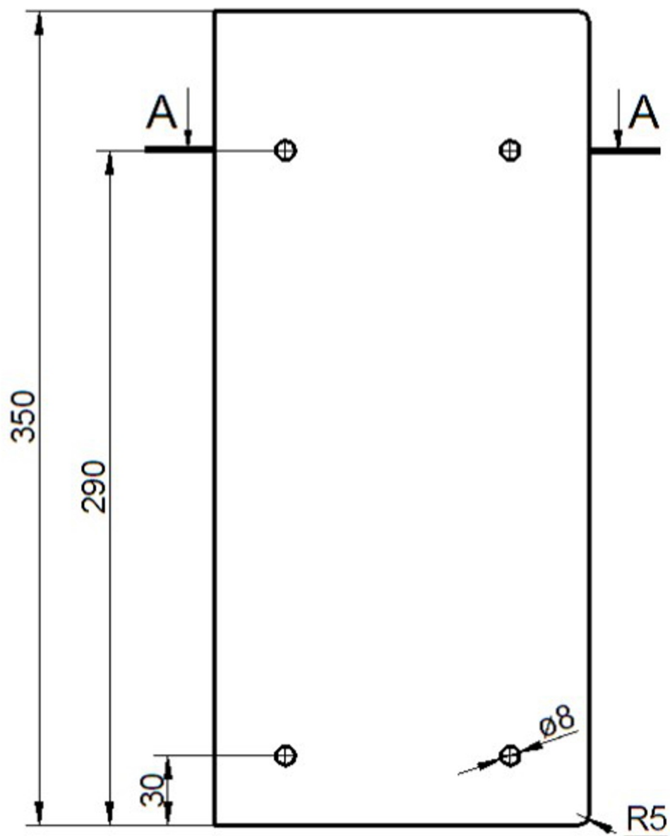
Rysunek 3. Ściana boczna
