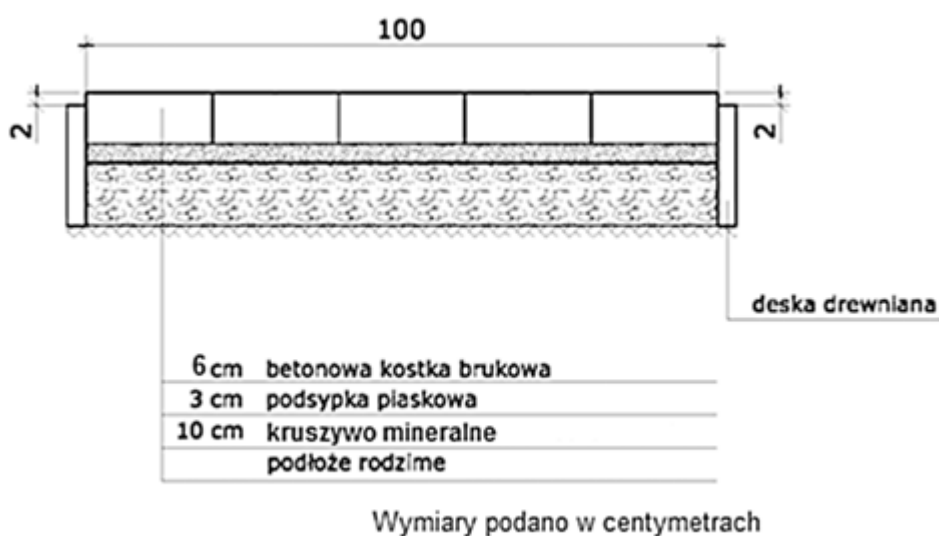
Rysunek 2. Przekrój poprzeczny nawierzchni chodnika
