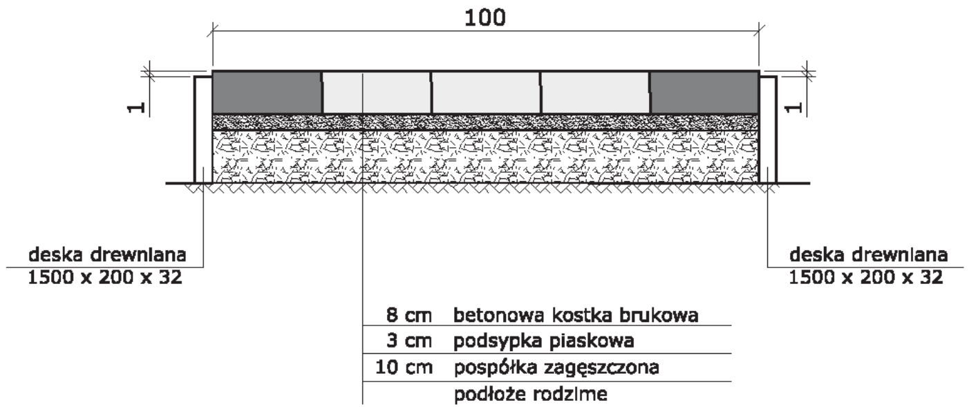
Rysunek 2. Przekrój poprzeczny nawierzchni z dwuteowej betonowej kostki brukowej.
