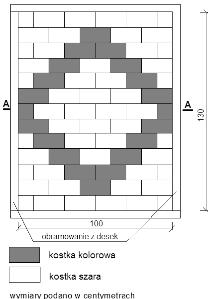
Rysunek 1. Widok fragmentu nawierzchni z betonowej kostki brukowej.
