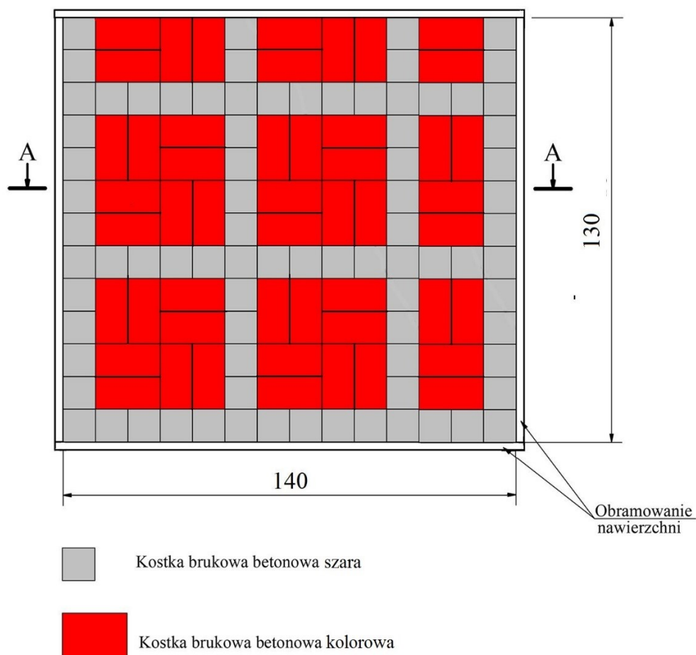
Rysunek 1. Rzut poziomy fragmentu nawierzchni do ułożenia
