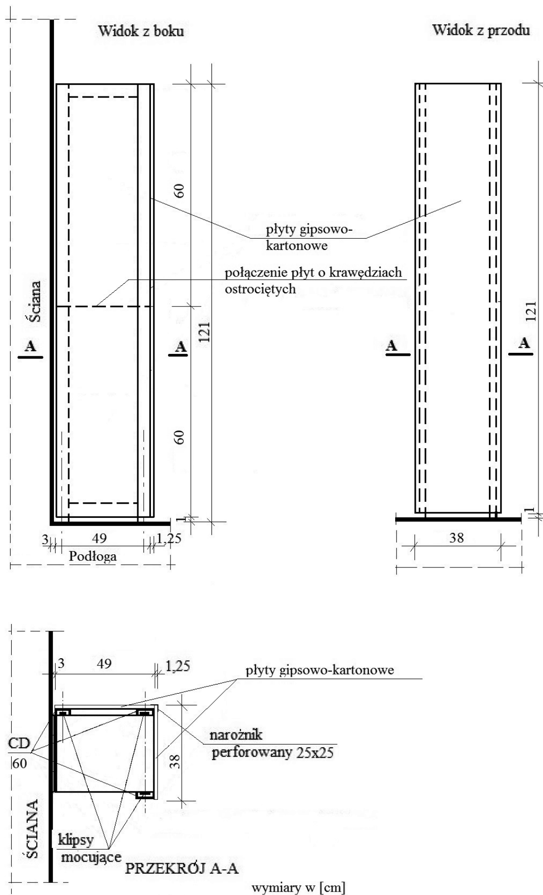
Rysunek 2. Schemat opłytywania
