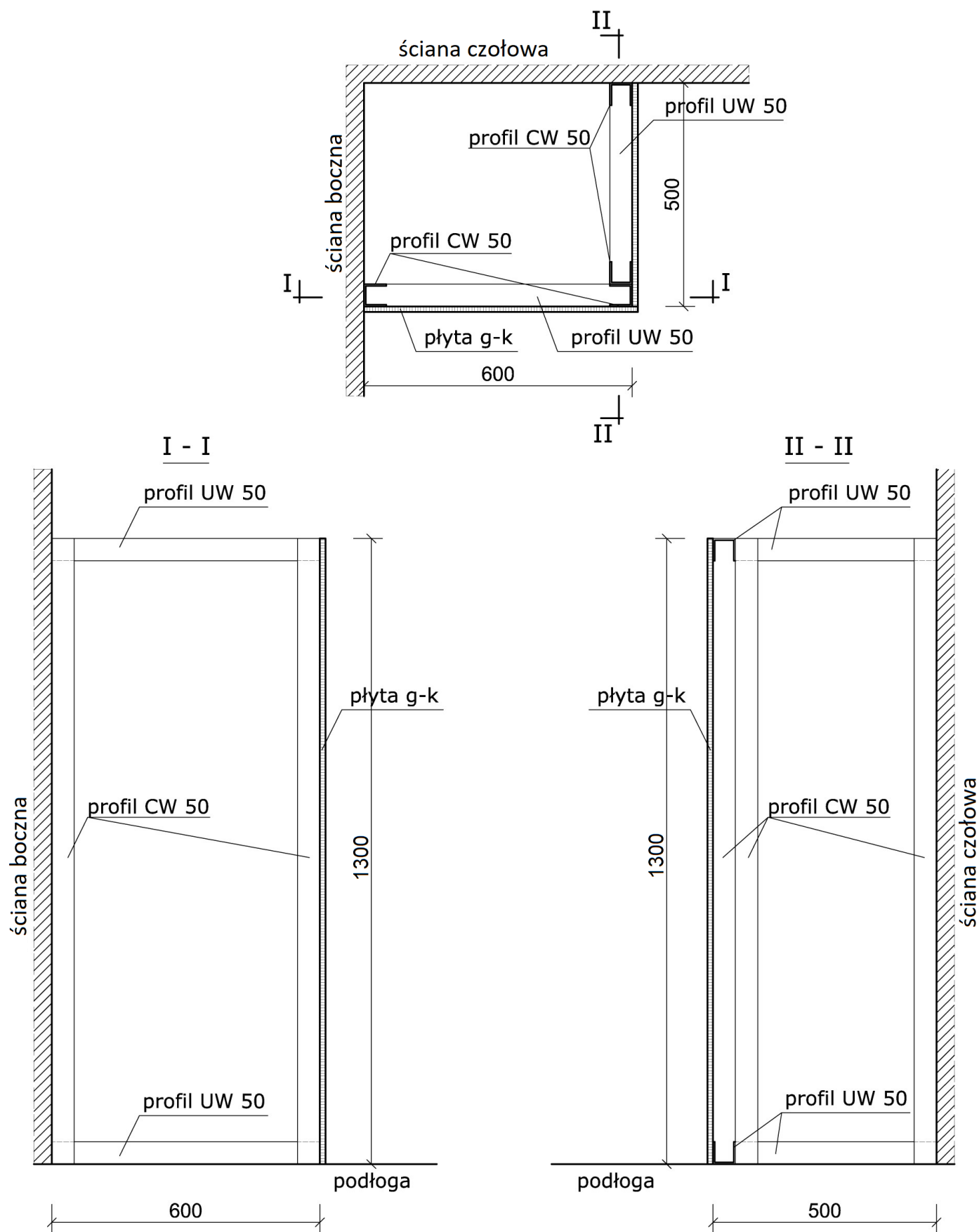
Rysunek. Konstrukcja zabudowy narożnika
