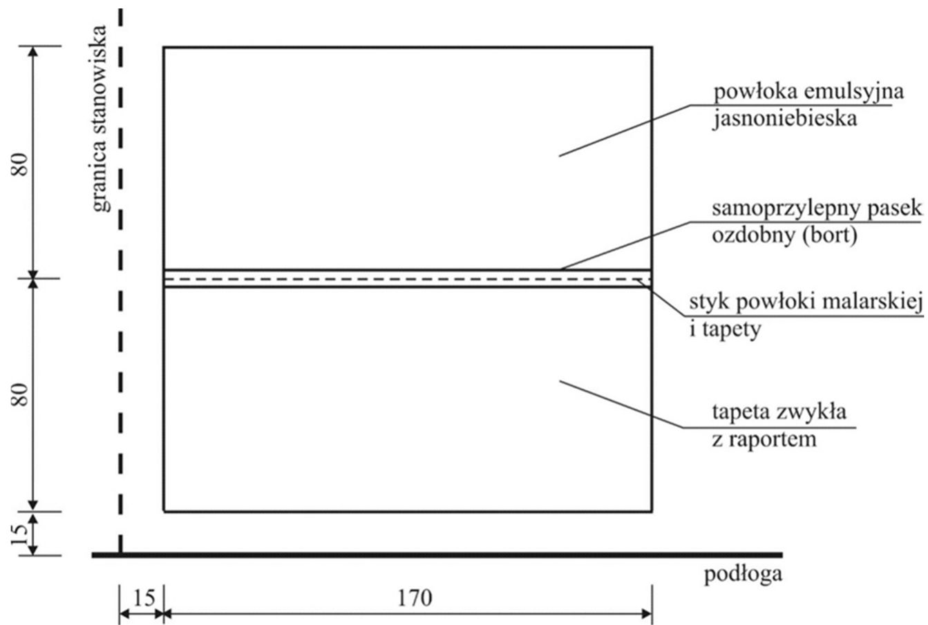
Rysunek 1. Widok wykończenia ściany
