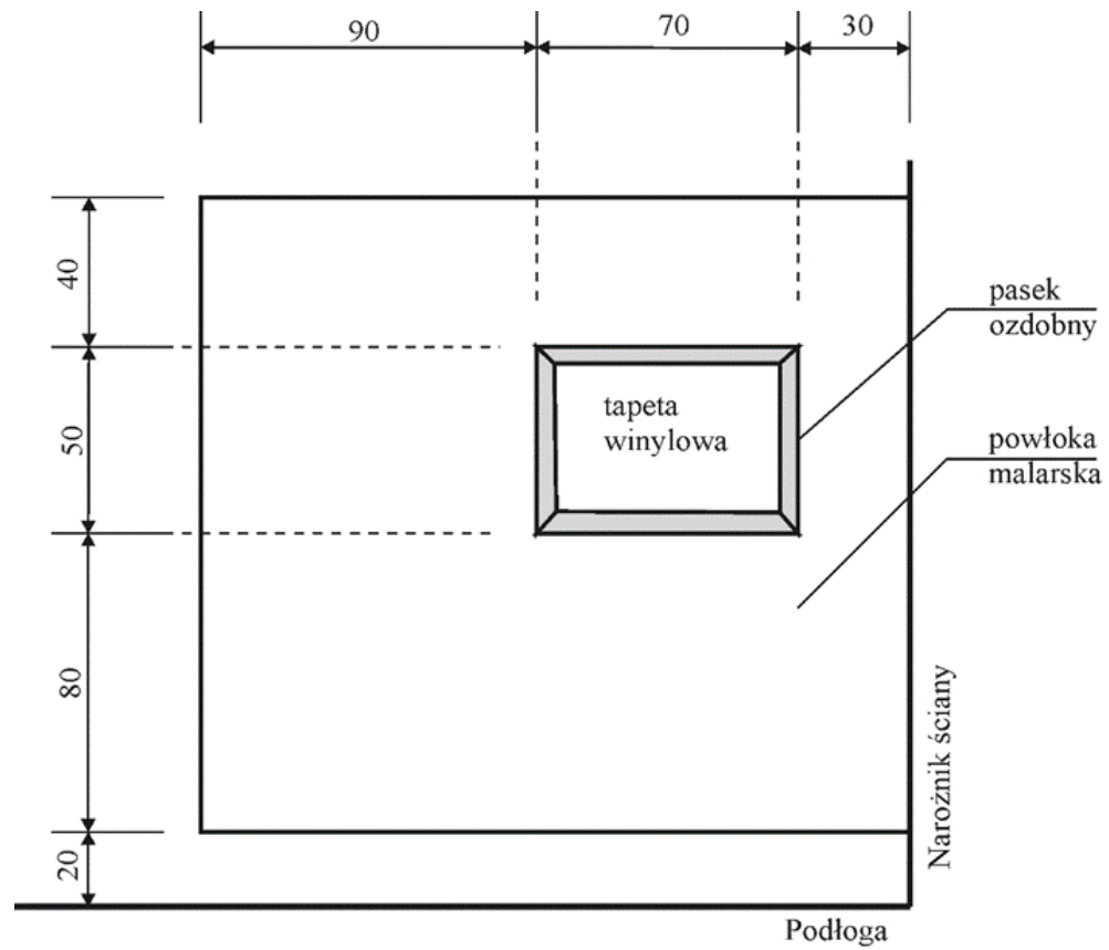
Rys. Widok wykończenia ściany
