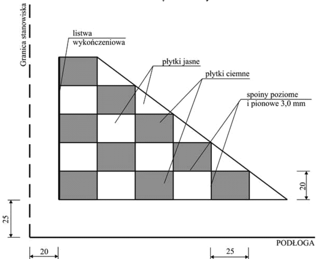
Widok okładziny ceramicznej
