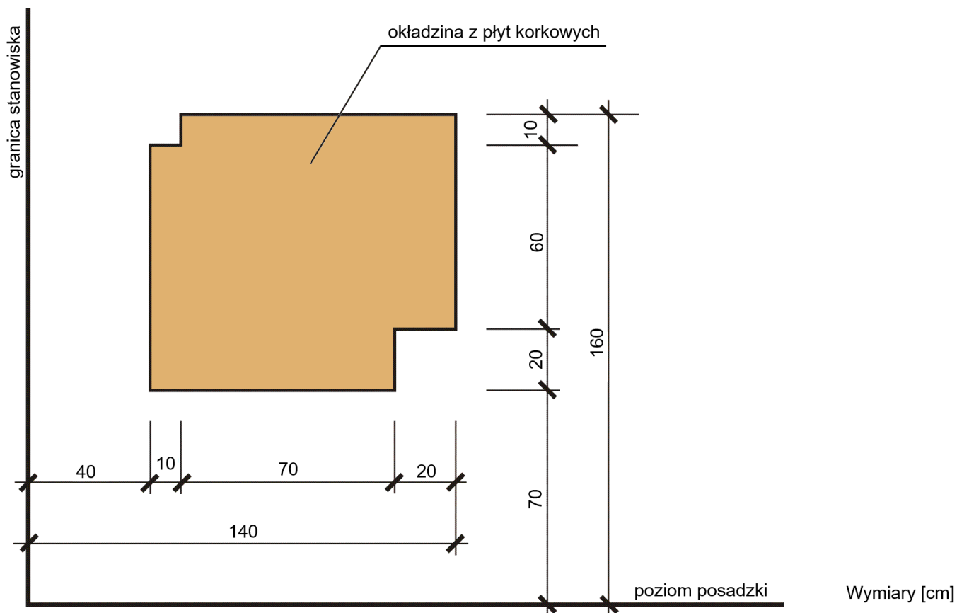
Rysunek. Fragment okładziny ściennej z płyt korkowych
