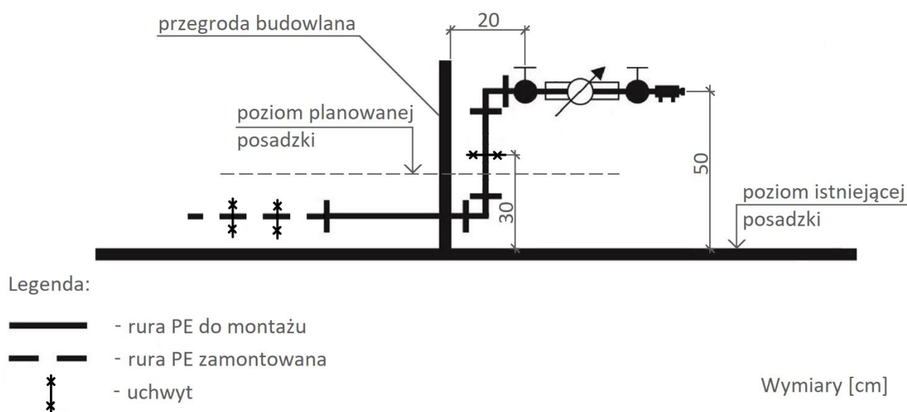
Rysunek. Schemat przyłącza wodociągowego
