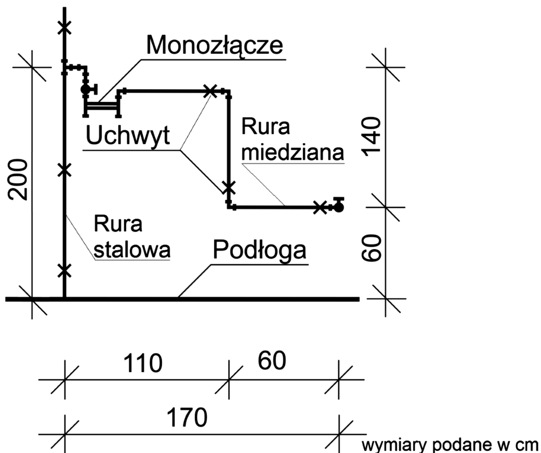
Schemat montażowy instalacji
