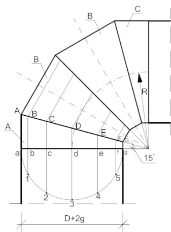
c) przekrój
