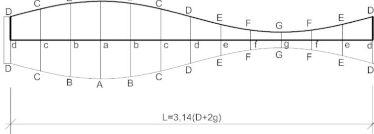
d) rozwinięcie
