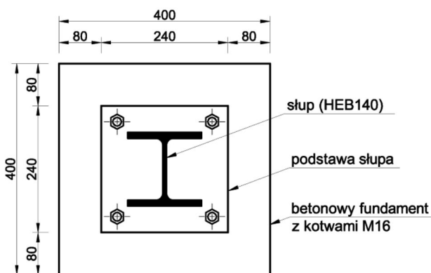
Fragment słupa na fundamencie - przekrój A - A:
