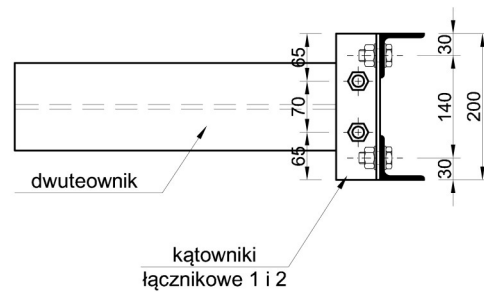
Rysunek 1 – Rysunek zestawieniowy (widok z góry, widoki boczne)
