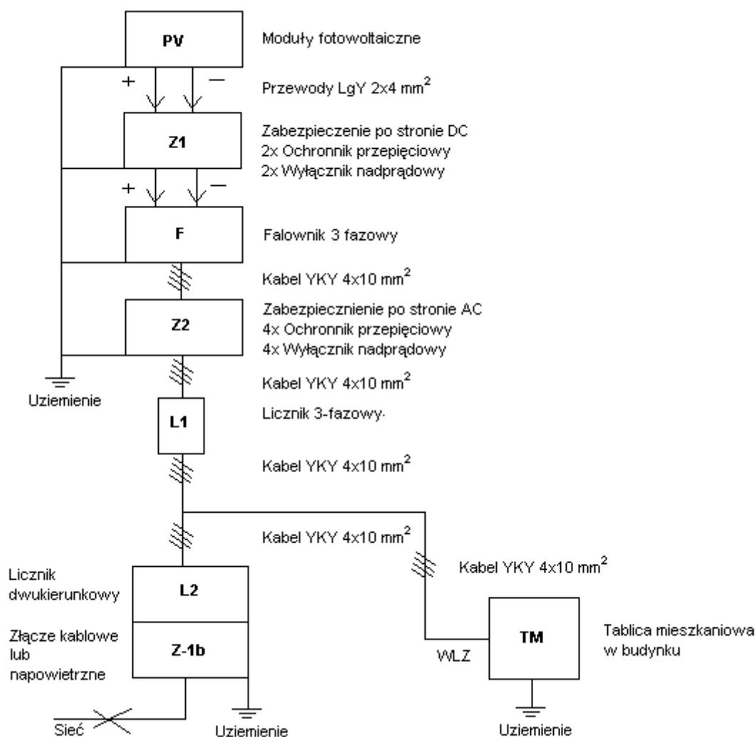
Przykładowy schemat blokowy instalacji fotowoltaicznej ON-GRID
