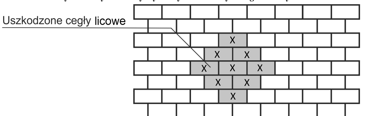
Rysunek wykonawczy wymiany uszkodzonych cegieł licowych
