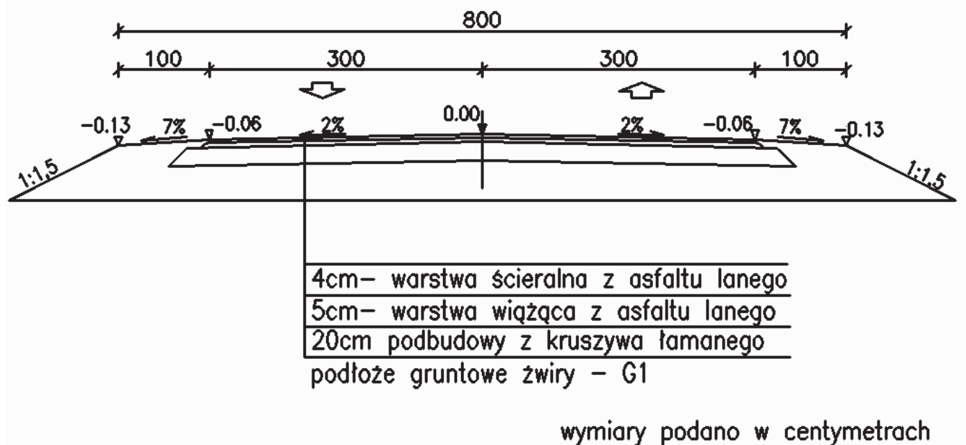
Przekrój poprzeczny drogi przed remontem PRZEKRÓJ POPRZECZNY
