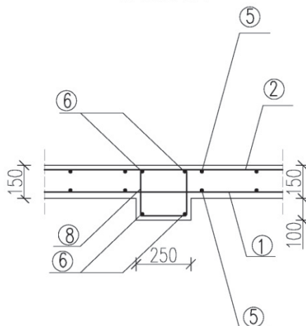
PRZĘKRÓJ C-C WIENIEC W2
