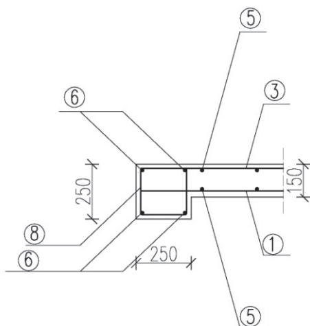
PRZĘKRÓJ A-A WIENIEC W2
