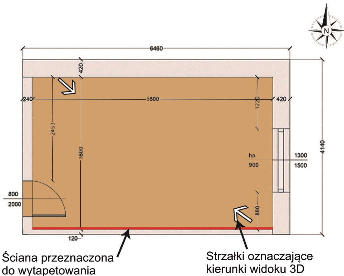
Rysunek 1. Rzut pokoju dziecięcego Wymiary podane w milimetrach
