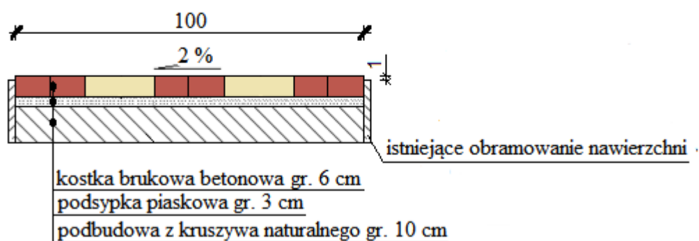
PRZEKRÓJ A - A [cm]
