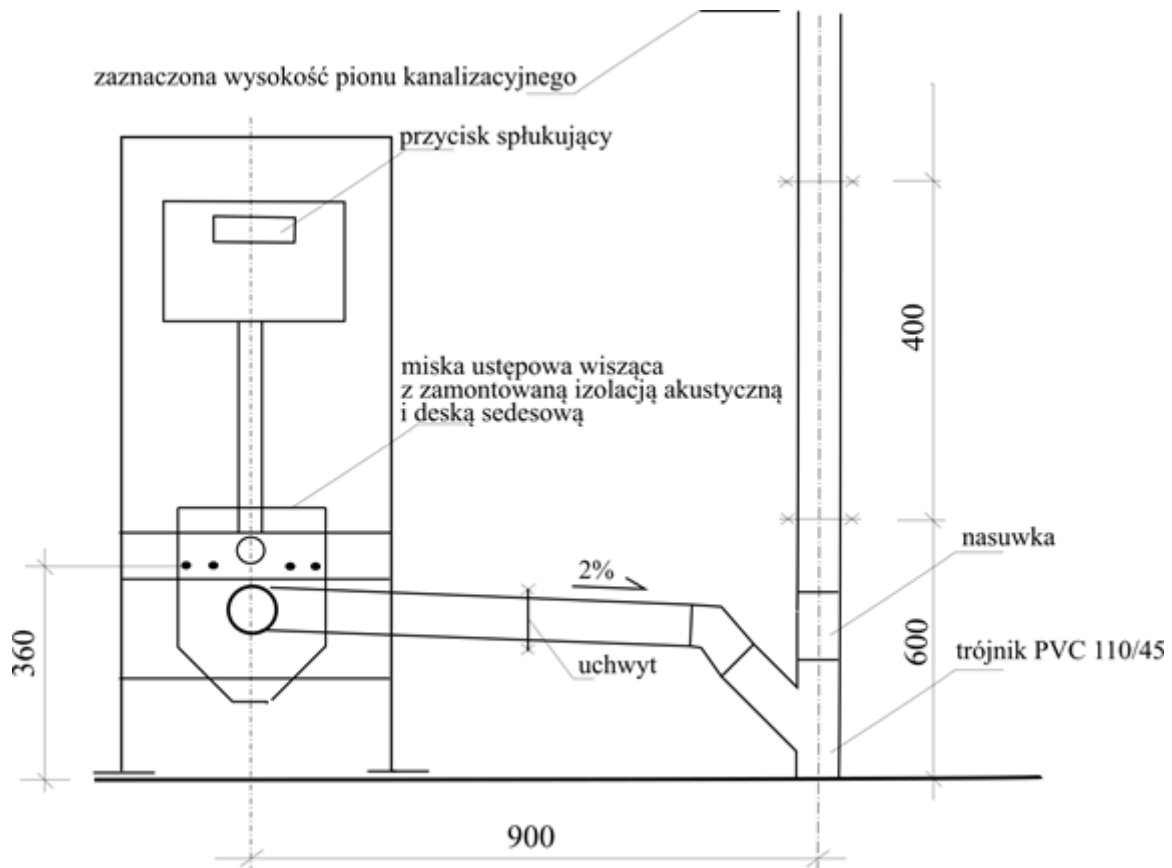
Schemat podłączenia podejścia kanalizacyjnego do stelaża miski ustępowej wiszącej (wymiary podane w mm)
