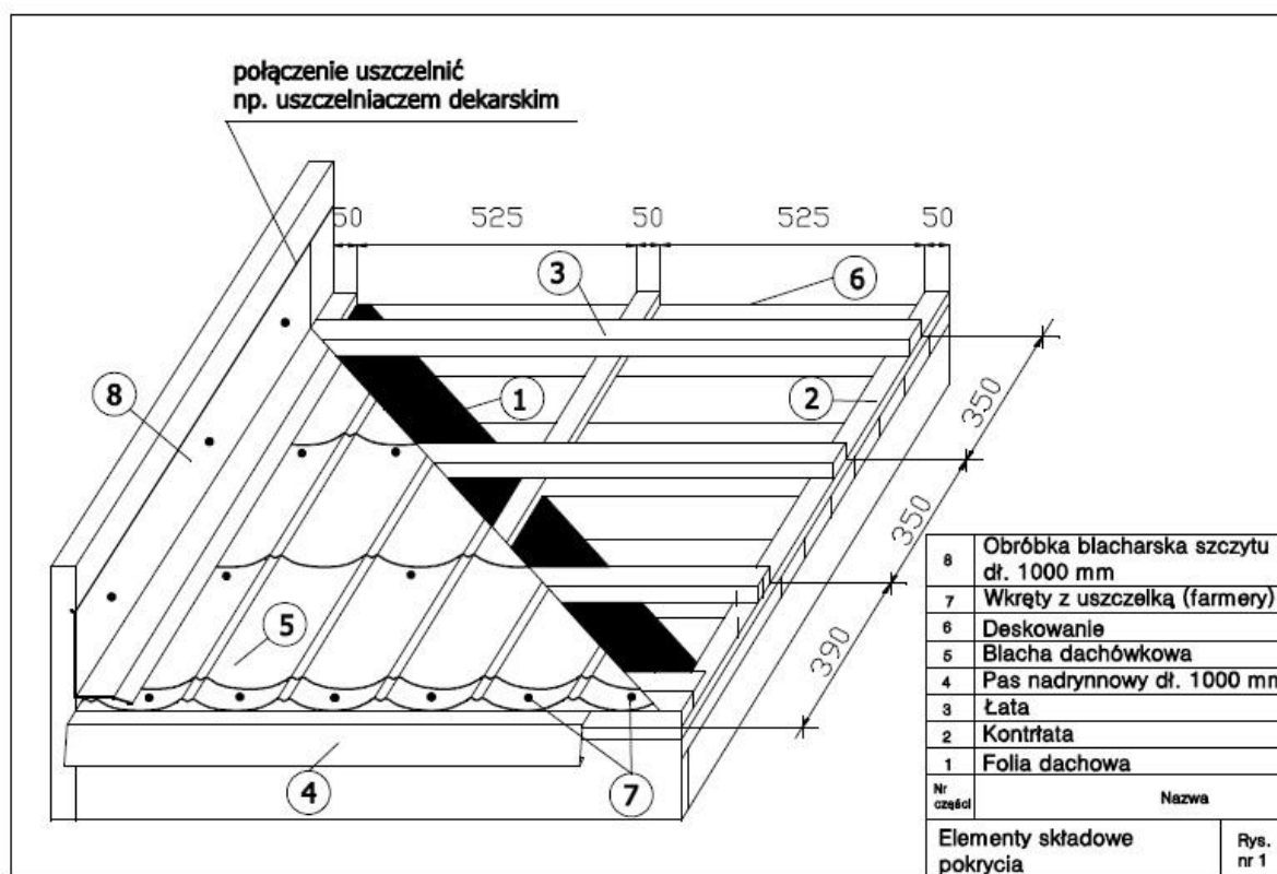
Rysunek 1. Schemat rozmieszczenia kontrłat i łat
