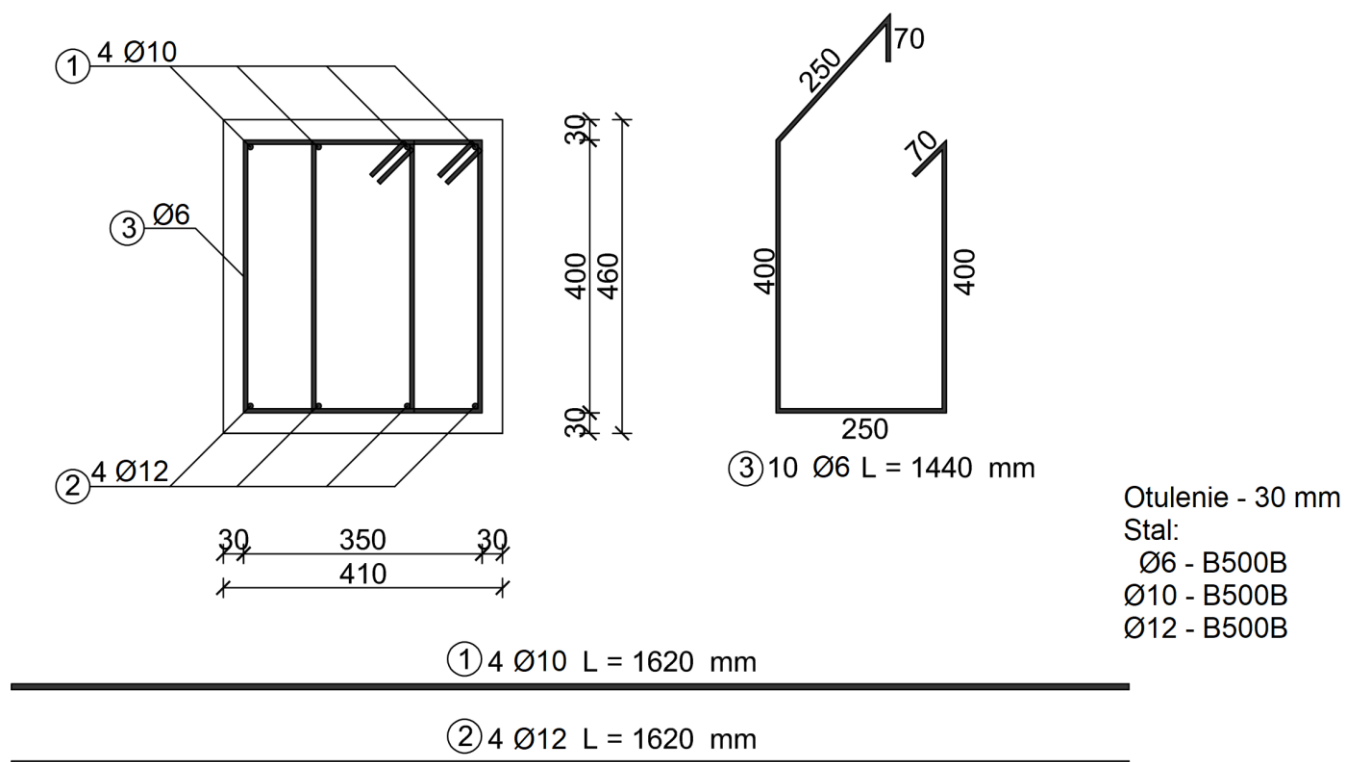
Rysunek 2. Przekrój A-A belki nadprożowej
