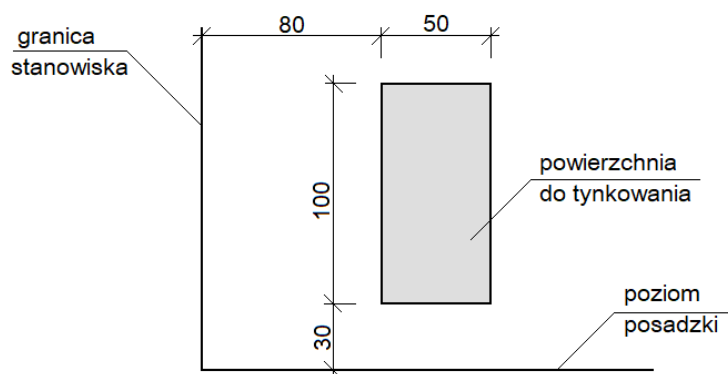
Rysunek 4. Usytuowanie tynku cienkowarstwowego mineralnego na stanowisku egzaminacyjnym (widok)
