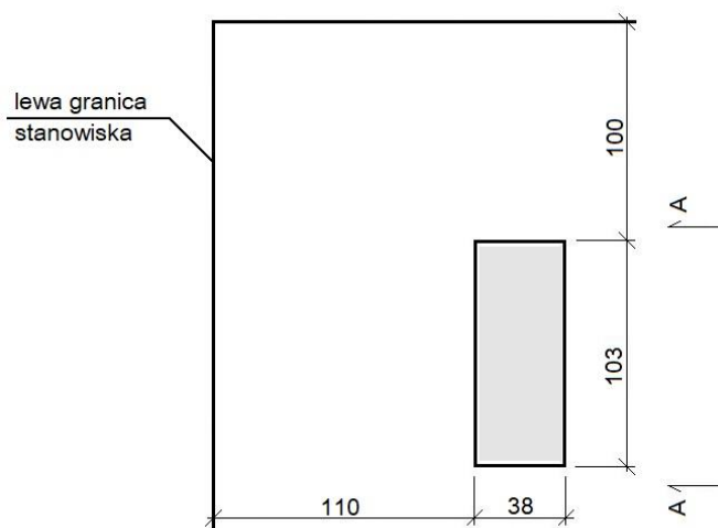
Rysunek 1. Usytuowanie fragmentu muru na stanowisku egzaminacyjnym (rzut)
