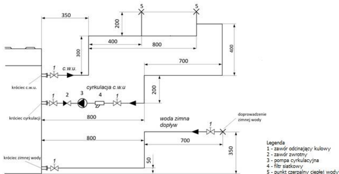
Rys.1 Schemat instalacji.
