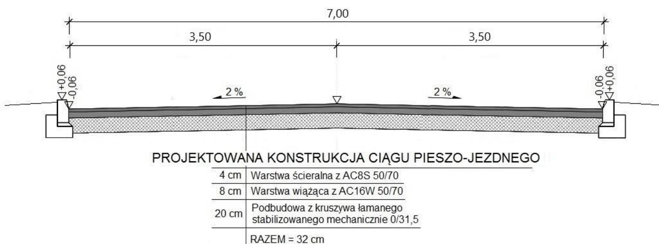
Przekrój normalny ciągu pieszo-jezdnego [ m ]
