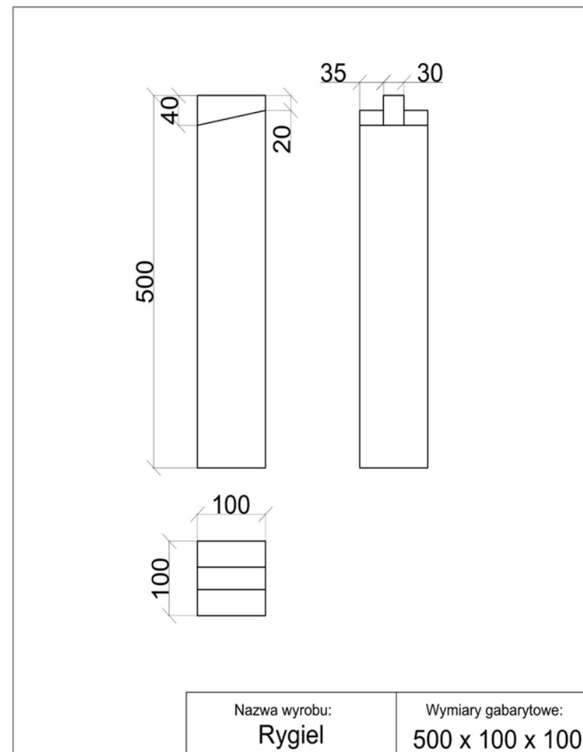
Rysunek 2. Rygiel
