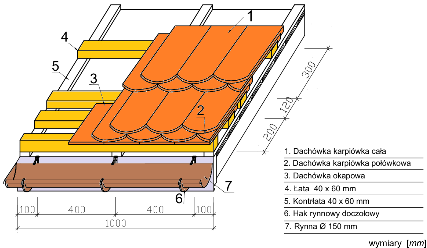
Rysunek 1. Elementy pokrycia dachowego
