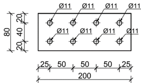
Rysunek 2. Blacha łącznikowa nr 3 (2 sztuki) – rozmieszczenie otworów montażowych
