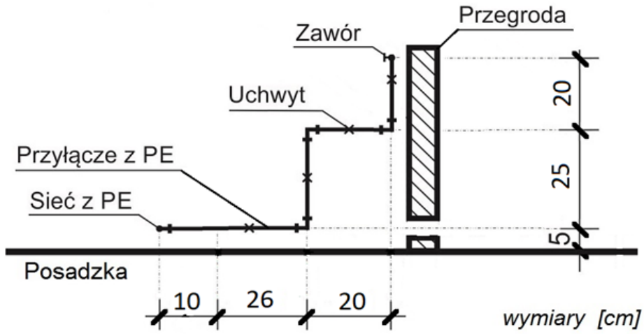
Rysunek 1. Przekrój pionowy przyłącza wodociągowego
